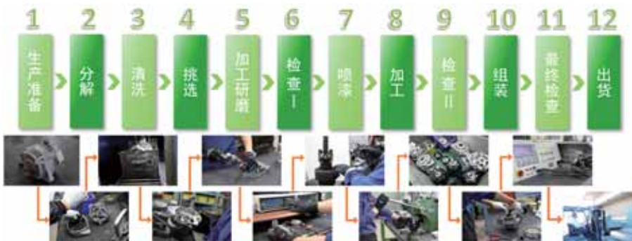
汽车零部件再造工艺流程图
